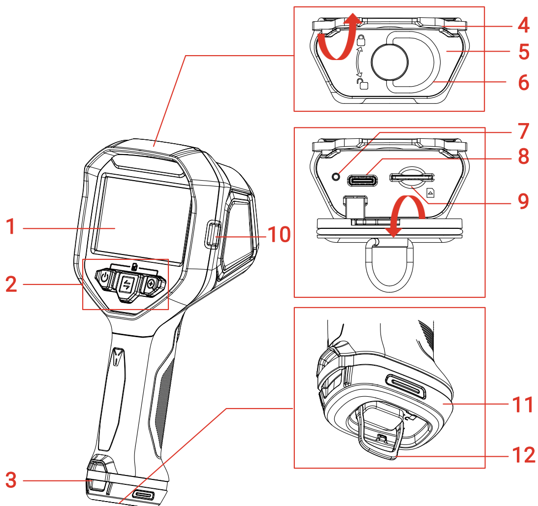
Figura 1-1 Aspecto (vista frontal)
