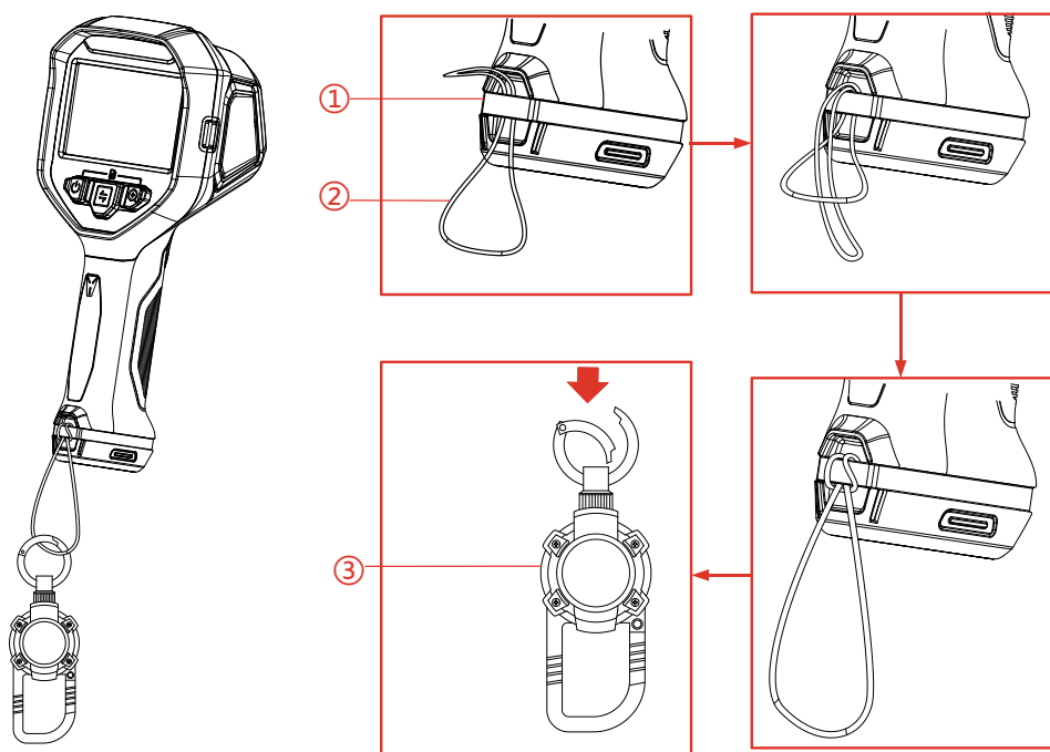
Figura 3-8 Colocar los cordones de seguridad
