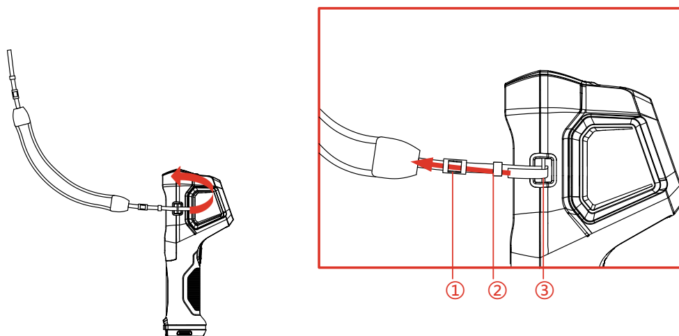
Figura 3-7 Colocar la correa para el cuello
